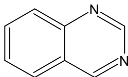
Chinazolina
