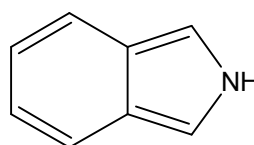
2H-izoindol
