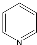
Pirydyna
