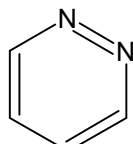
Pirydazyna
