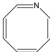
Azocyna
