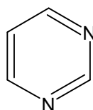
Pirymidyna
