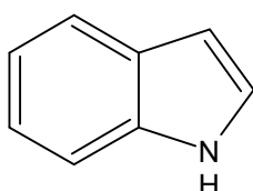
Indol
