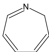
1H- azepina
