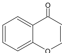
Hromon
