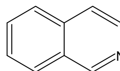
Izochinolina
