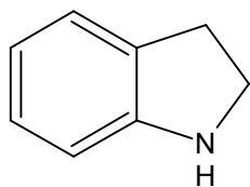
Indolina
