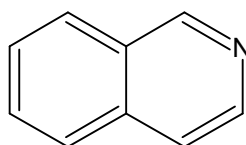
Cynnolina
