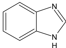
Benzimidazol
