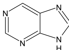
Puryna
